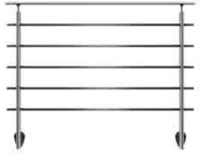
PS 201 ALUMINIUM TROPFEN Seitenmontage 5 Aluminiumstäbe, 2 Pfosten tropfenförmig, 1.500 mm, 1 Stck. Art.-Nr. 0196531
