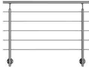
PS 011 ALUMINIUM RUND Seitenmontage, 5 Edelstahlstäbe, 2 Pfosten rund, 1.500 mm, 1 Stck. Art.-Nr. 0196412
